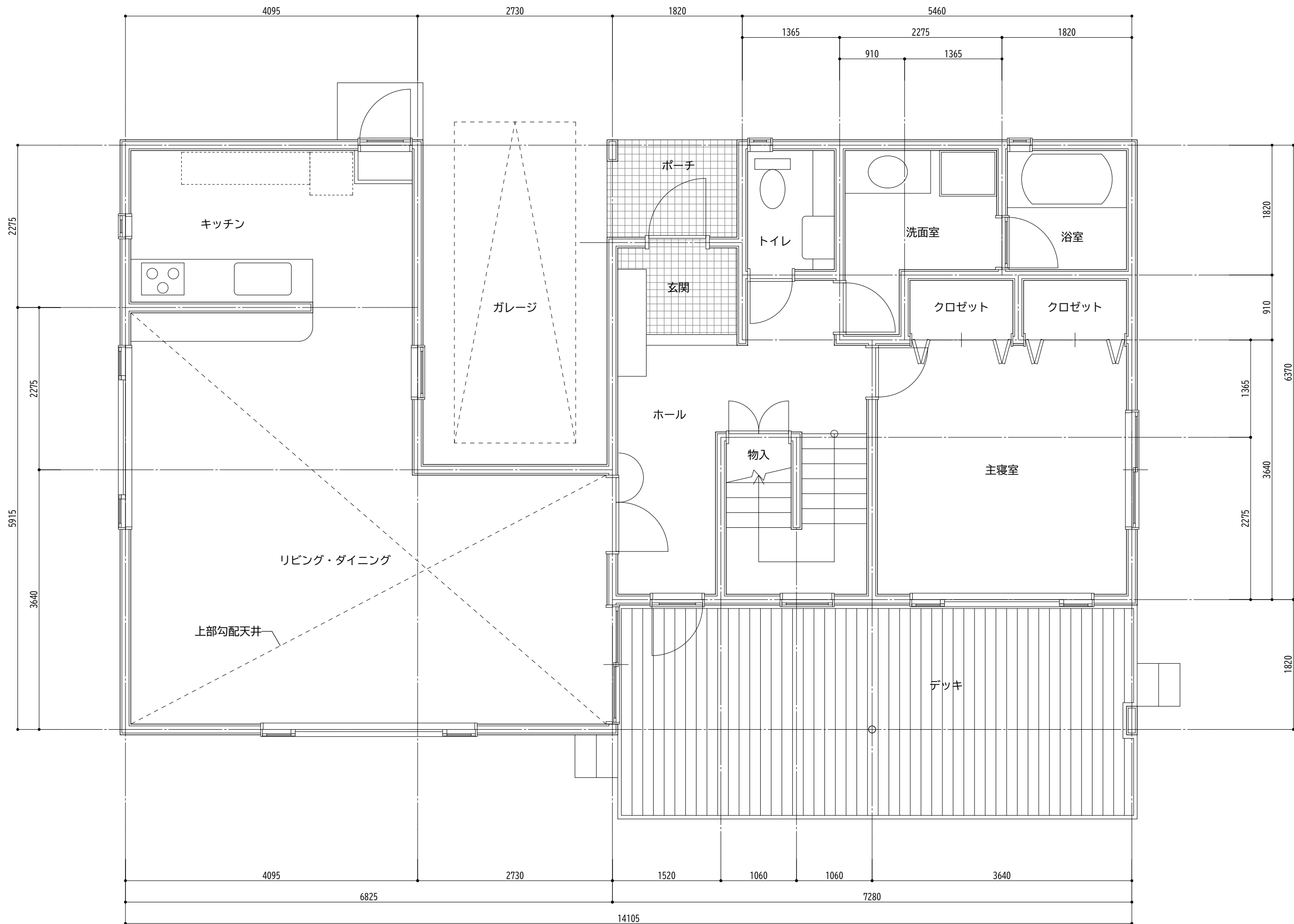
1階平面詳細図
